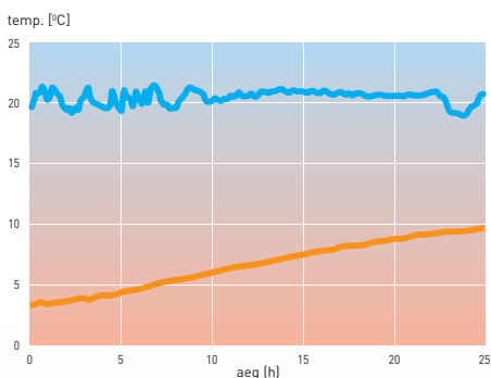
Roogade temperatuuritõus termokonteineris, täislaadimisel — algtemperatuur 2,3°C — keskkonna temperatuur 20°C
